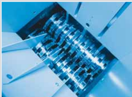
Accessoire HSM DuoShredder 5540.2 : précompacteur électro-hydraulique dans la goulotte avec dispositifs de sécurité en cas de surcharge intégrés pour matériaux particuliers
